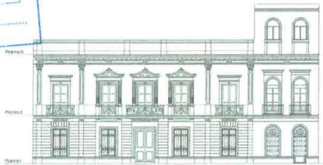
Ampliación propuesta. Volúmenes 01 y 02.
