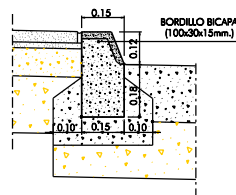
DETALLE "B" BORDILLO DE CONFINAMIENTO SIN ESCALA
