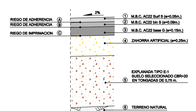
DETALLE "2" SECCION TIPO PAQUETE DE FIRME EN CALZADA SIN ESCALA
