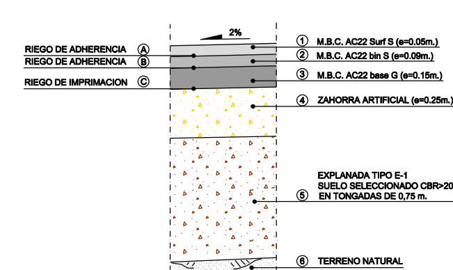
DETALLE "2" SECCION TIPO PAQUETE DE FIRME EN CALZADA SIN ESCALA
