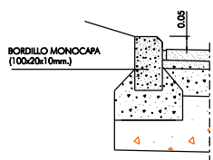
DETALLE "B" BORDILLO DE CONFINAMIENTO SIN ESCALA
