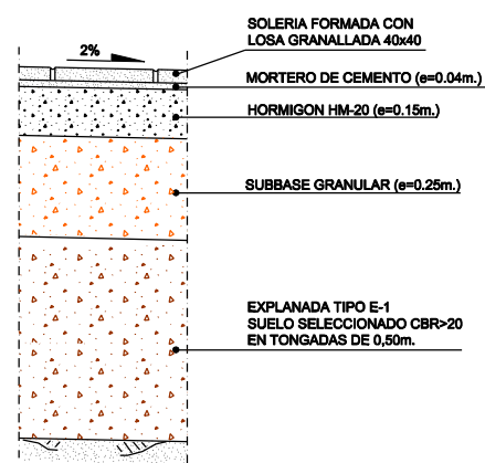
DETALLE "1" SECCION TIPO ACERADOS SIN ESCALA
