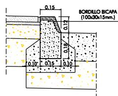
DETALLE "B" BORDILLO DE CONFINAMIENTO SIN ESCALA
