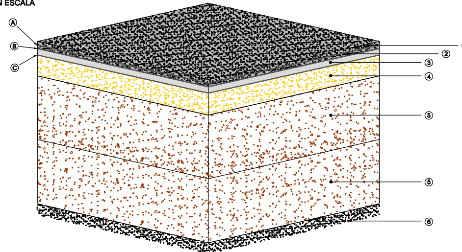
DETALLE "2" PERSPECTIVA DEL PAQUETE DE FIRME EN CALZADA SIN ESCALA
